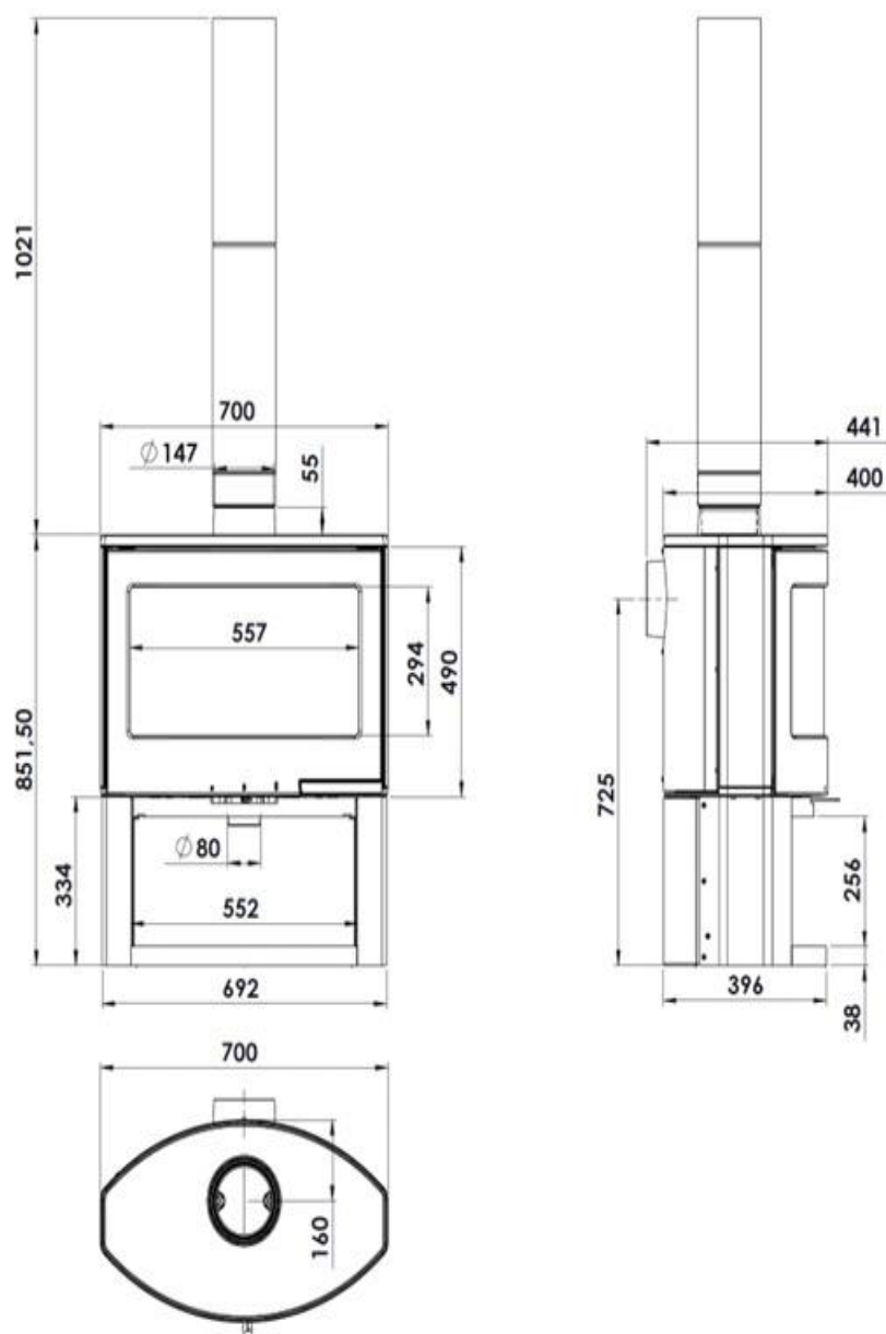
Figura n°1 - Dimensioni in mm dell'apparecchio Dublin Star / Bristol Star
