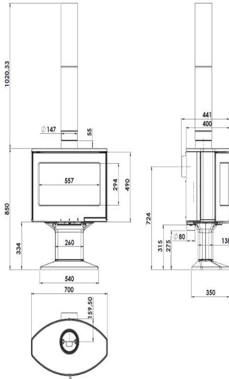
Figura n°1 - Dimensioni in mm dell'apparecchio Tarbes Star
