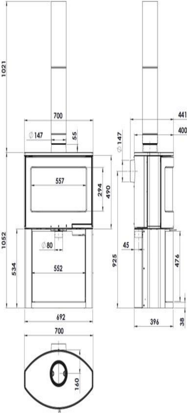
Figura n°2 - Dimensioni in mm dell'apparecchio Bera
