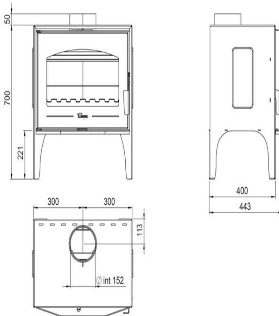
Figura n°1 - Dimensioni in mm dell'apparecchio Calpe.
