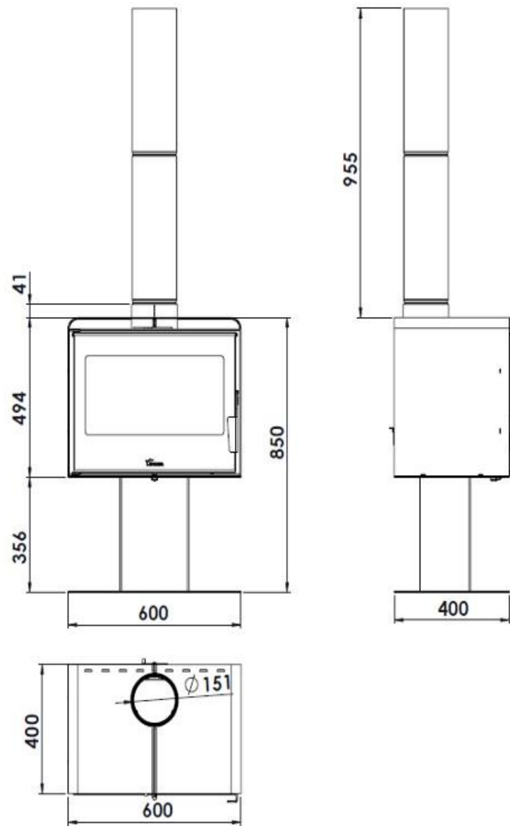
Figura n°1 - Dimensioni in mm dell'apparecchio serie Ocean/Atlantic 600
