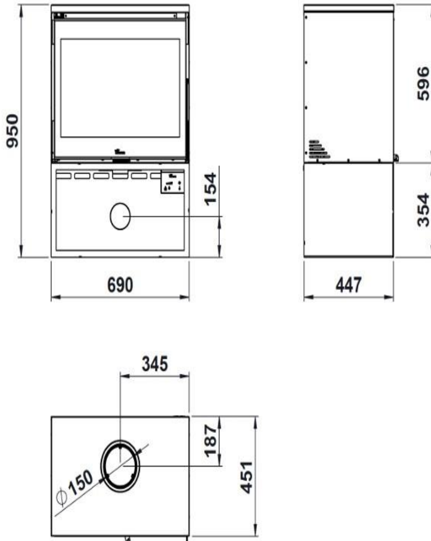
Figura n°1 - Dimensioni in mm dell'apparecchio ROMA 700
